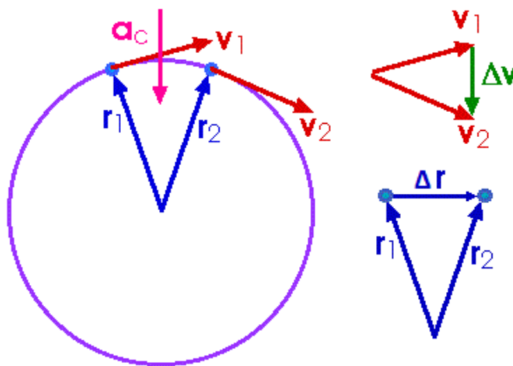
Figur 3.10: Utledning av sentripetalakselerasjon
