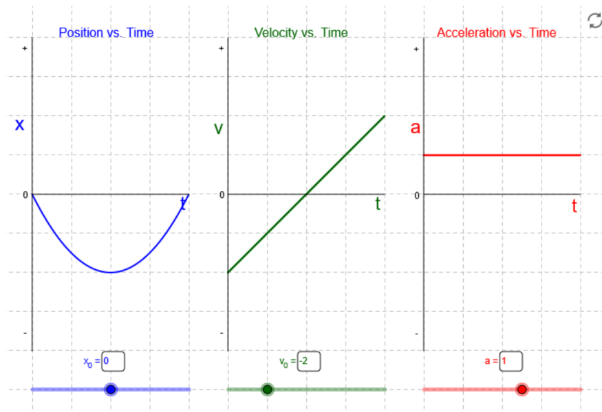
Figur 3.3: Eksempel på posisjon, hastighet og akselerasjonsgraf hvor akselerasjonen er konstant
